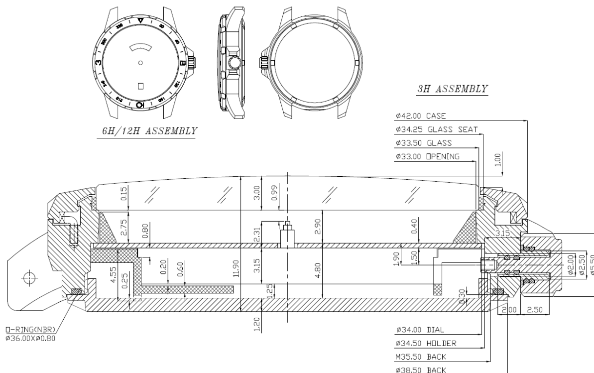
Чертеж корпуса.
